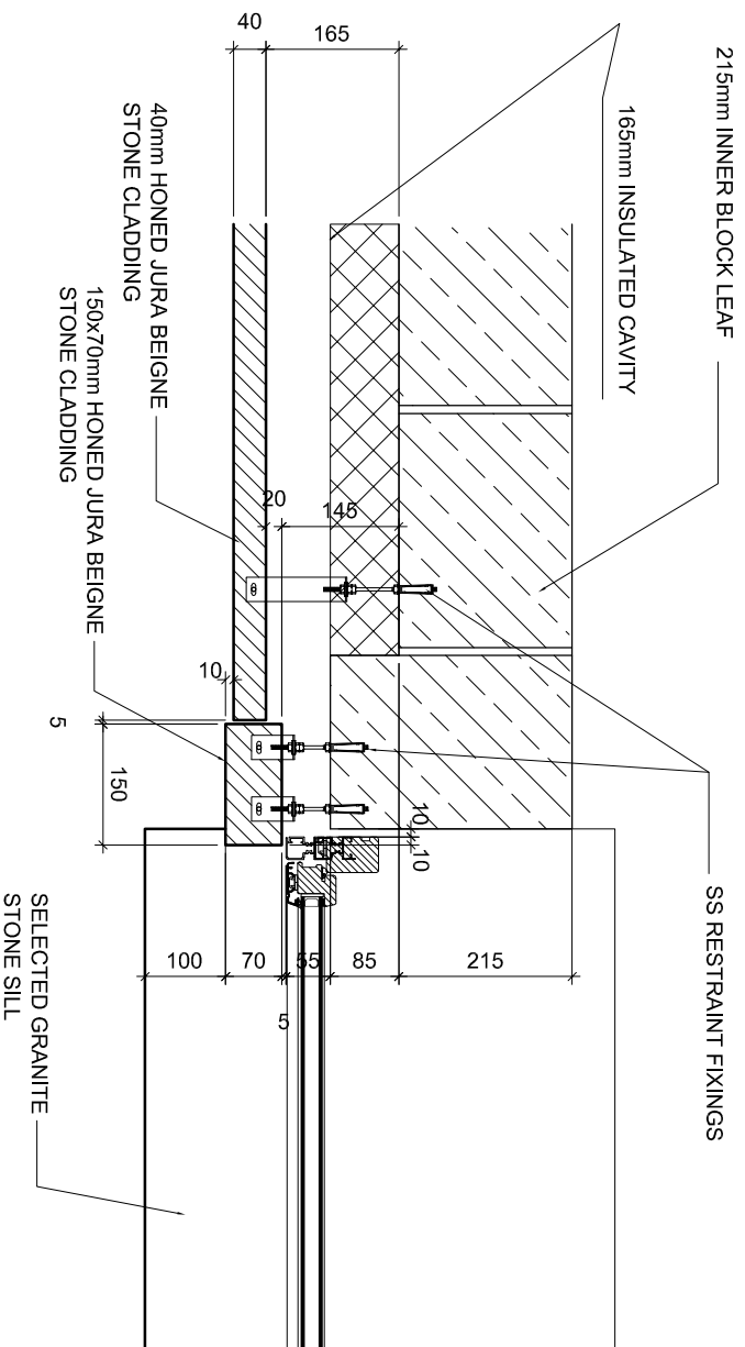
DETAIL 18 SCALE: 1:10
