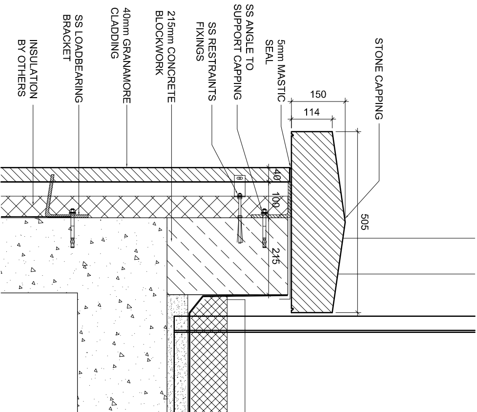
DETAIL 14 SCALE: 1:10
